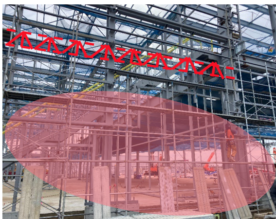
①梁枠を設置するための足場を設置
